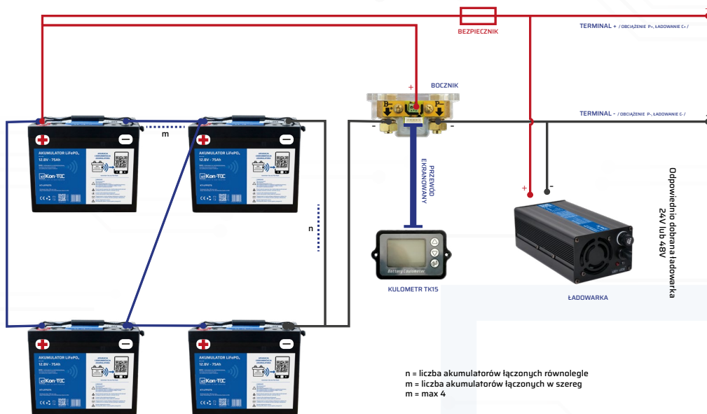
Rys.5. Schemat szeregowo-równoległego połączenia akumulatorów
