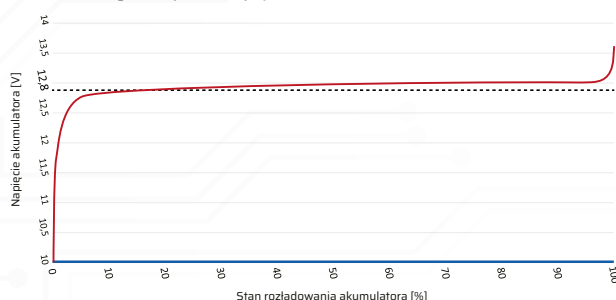
Rys. 8 Spadek napięcia akumulatora, rozładowanie 1C
