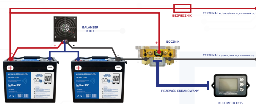
Rys.3. Schemat szeregowego połączenia akumulatorów
