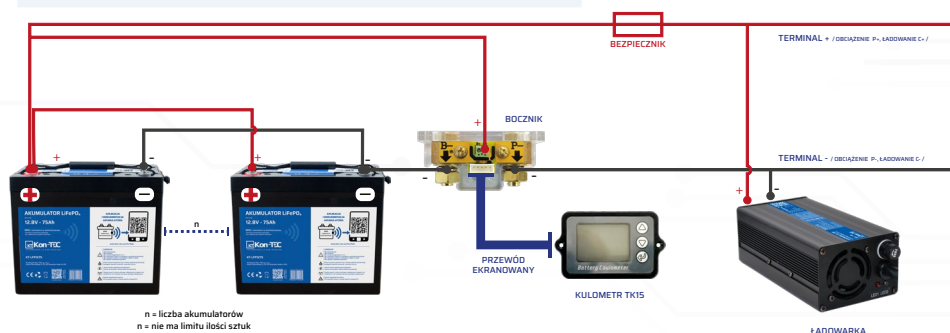
Rys.4. Schemat równoległego połączenia akumulatorów
