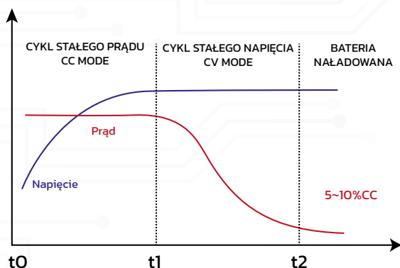
Rys.6. Cykle ładowania dla akumulatorów litowo-jonowych
