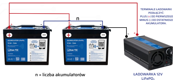
Rys.2. Schemat podłączenia pojedynczego akumulatora
